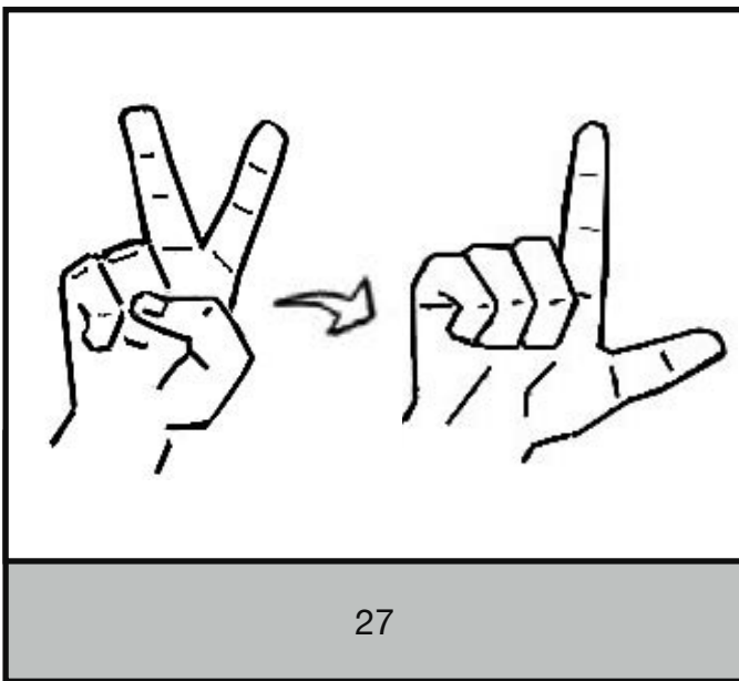
සියක් දහස 100,000
